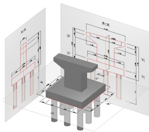
三面図コマンドによる構造物の3Dモデル化
